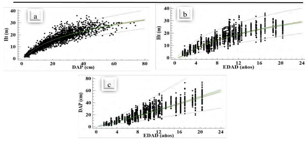
Figura 2. Modelos predictivos de la altura total y el DAP en árboles de C. odorata en SAF, Pérez Zeledón, Costa Rica, 2019: a) Ht en función DAP, b) Ht en función a la EDAD, c) DAP en función a la EDAD.
