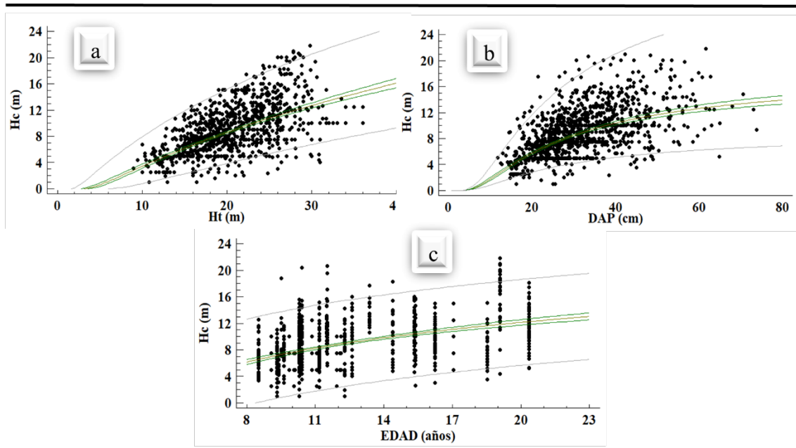
Figura 3. Modelos predictivos de la altura comercial de C. odorata en SAF, Pérez Zeledón, Costa Rica, 2019: a) en función del Ht, b) en función del DAP, c) en función de la EDAD.
