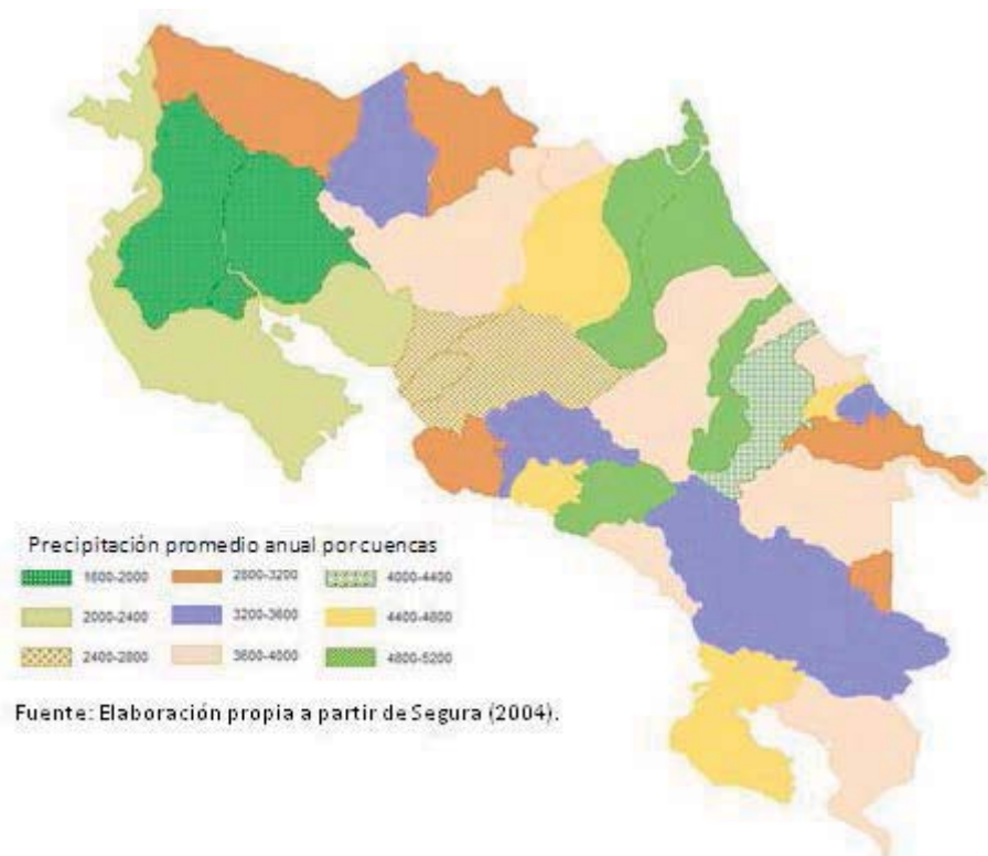
Mapa 1. Cuencas de Costa Rica y distribución de precipitaciones anuales por cuenca.
