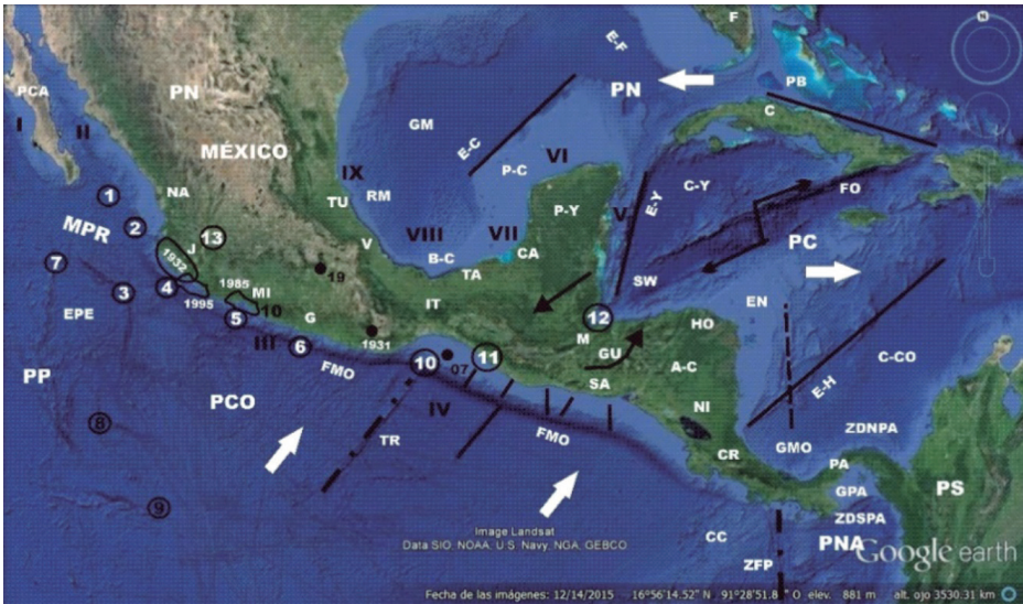
Figura 1. Esquema tectónico
