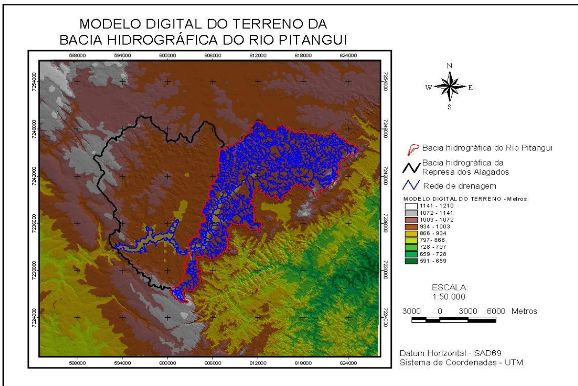
Figura 02 – Modelo Digital do Terreno da Bacia hidrográfica do rio Pitangui.
