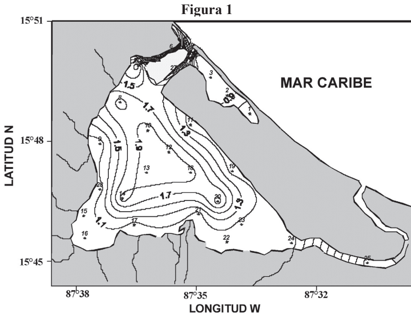
Posición de las estaciones hidrográficas y batimetría (m).
